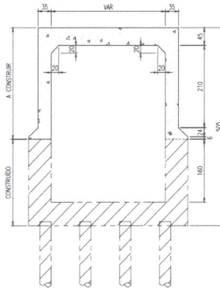
CORTE A-A ESC. 1:50
